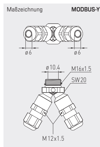
Maßzeichnung SF-M
