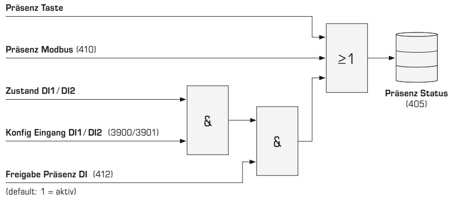
Abb. 028 Präsenzänderung
