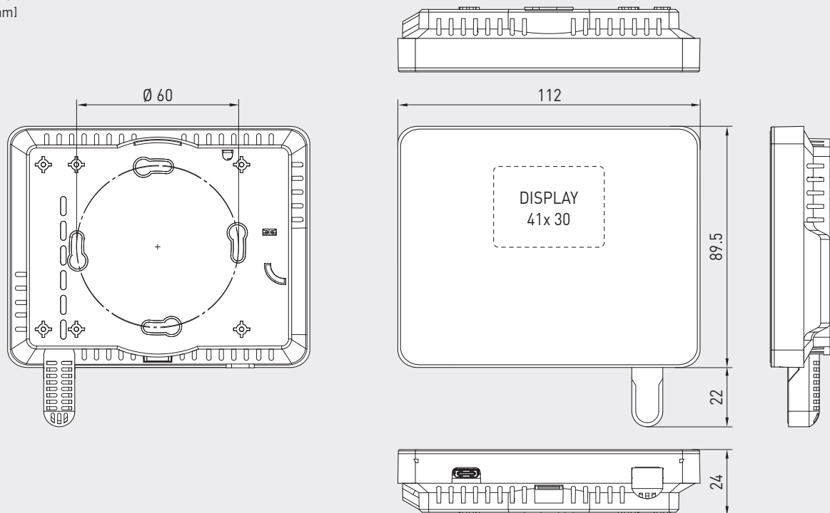
Maßzeichnung Aufputz-Variante Iduna 3 [mm]
