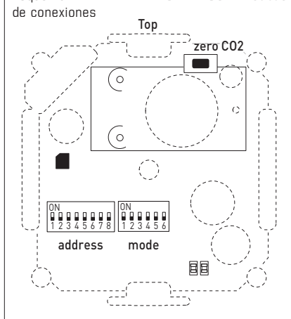
Esquema de conexiones FSFTM - CO2 - Modbus
